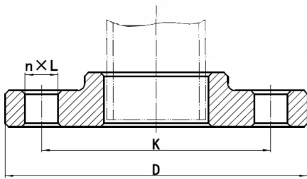
图4-4 平面（FF）带颈平焊钢制管法兰
