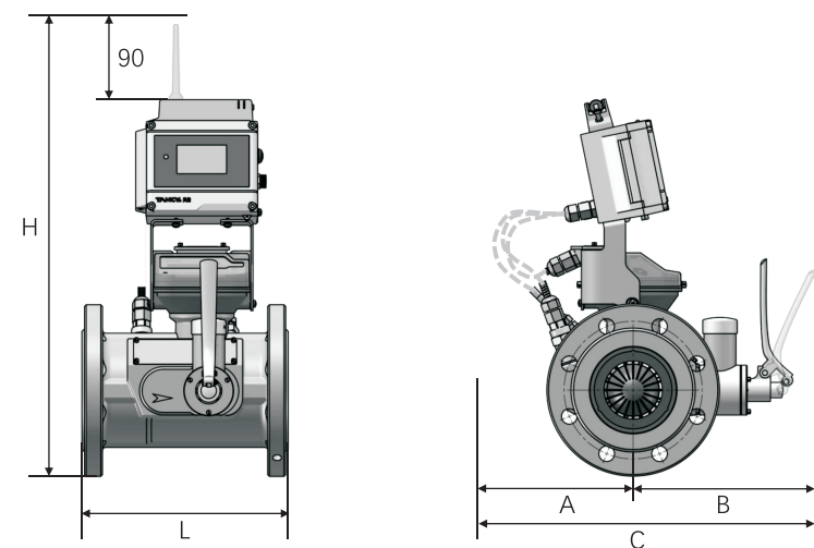
图3-5 TBQM-□/TFC-V
