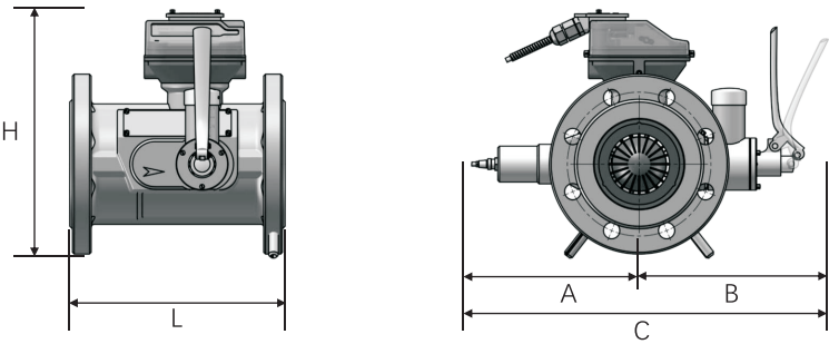
图3-1 TBQM-□基本型
