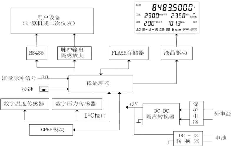
图1 修正仪工作原理框图
