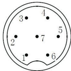
图5 航空插座
