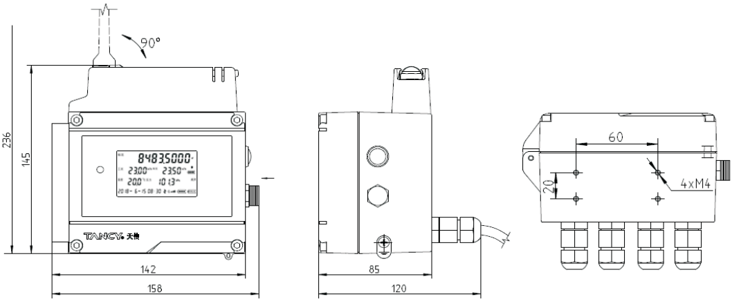
图2 外型尺寸图
